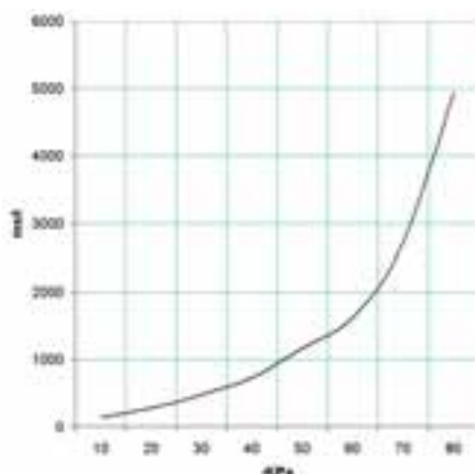
Temps d'évacuation (ms/l = s/m³) aux différents niveaux de vide (-Kpa)
