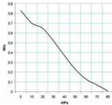
Débit d'air (NI/s) aux différents niveaux de vide (-Kpa)
