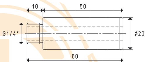
Silencieux art. SSX 1/4" sur M3
