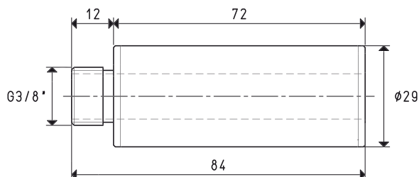
Silencieux art. SSX 3/8" sur M7
