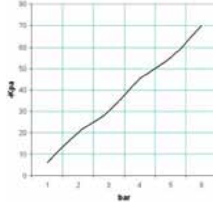
Consommation d'air (Nm 3 /s) aux différentes pressions d'alimentation (bar)
