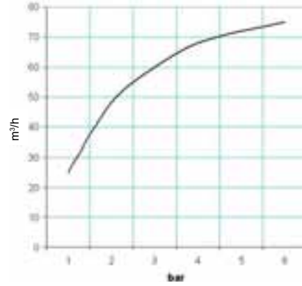
Quantité d'air soufflée (m 3 /h) aux différentes pressions d'alimentation (bar)
