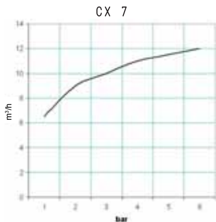
Quantité d'air soufflée (m 3 /h) aux différentes pressions d'alimentation (bar)
