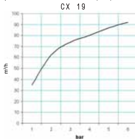
Quantité d'air soufflée (m³/h) aux différentes pressions d'alimentation (bar)
