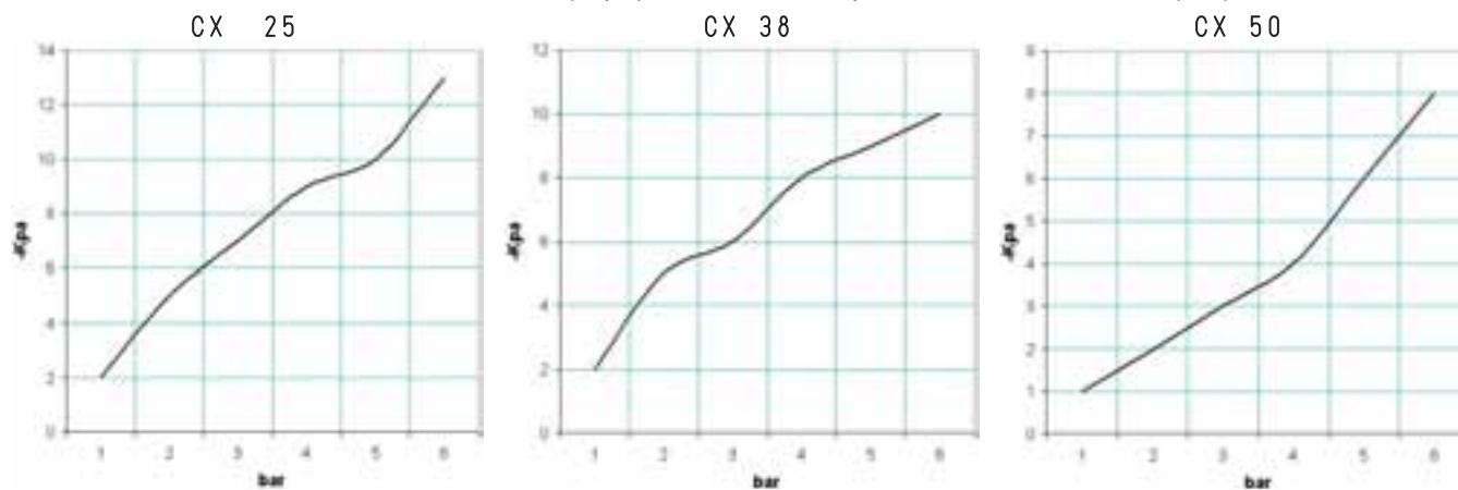
Consommation d'air (NI/s) aux différentes pressions d'alimentation (bar)
