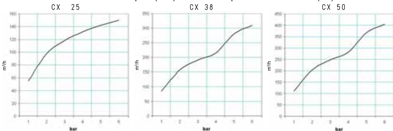
Quantité d'air soufflée (m³/h) aux différentes pressions d'alimentation (bar)
