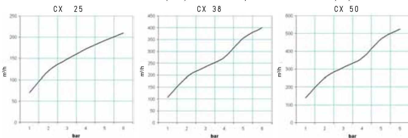
Niveau de vide (-Kpa) aux différentes pressions d'alimentation (bar)
