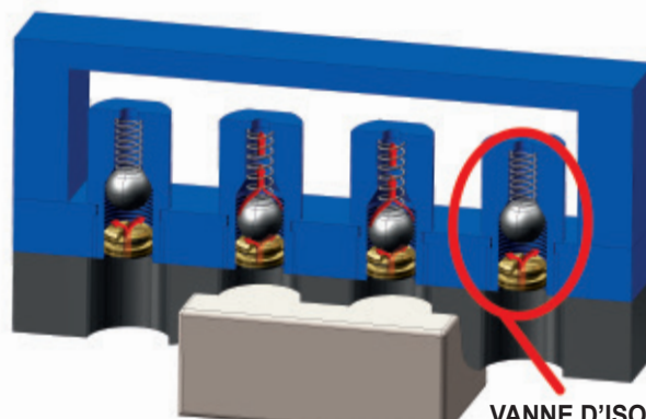
VANNE D'ISOLEMENT AUTOMATIQUE
